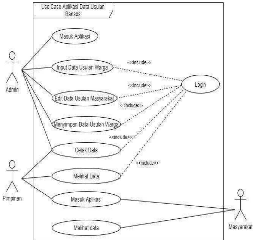
Gambar 1. Use Case Diagram Aplikasi Data Usulan Bansos
