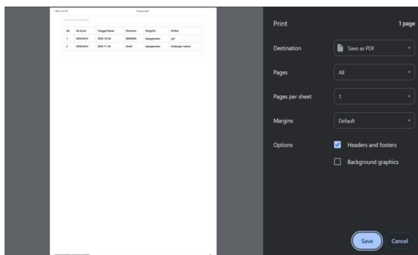
Gambar 15. Cetak
