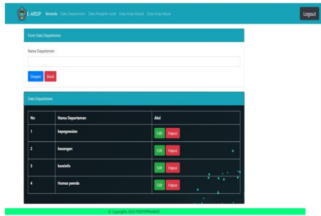
Gambar 8. Data departemen
