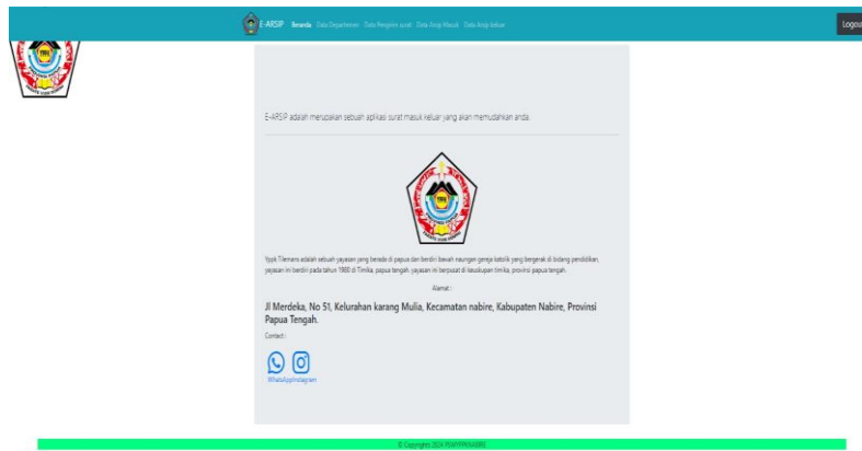
Gambar 7. Beranda
